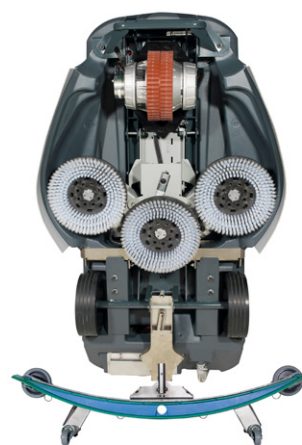
650 mm Arbeitsbreite
