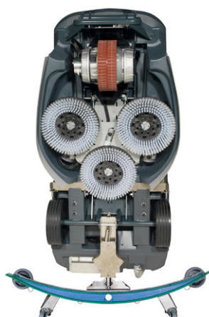
850 mm Arbeitsbreite
