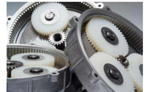
Langlebiges Planetengetriebe
